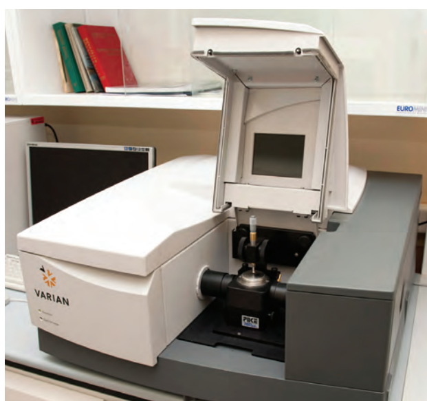
ИК-Фурье спектрометр Varian 640-IR
