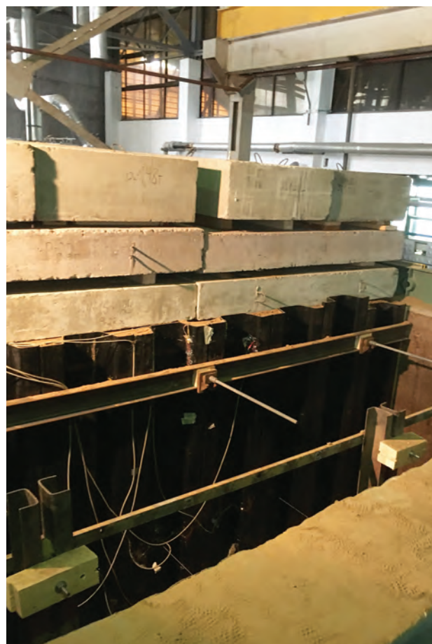
Грунтовый лоток
