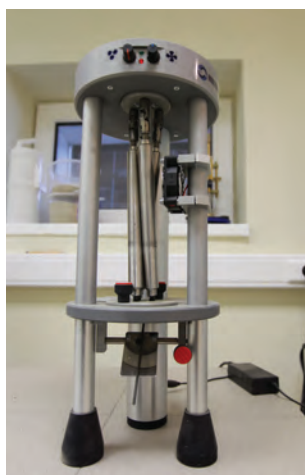
Установка для определения пластичности на границе раскатывания
