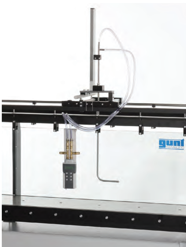
Трубка Пито–Прандтля
