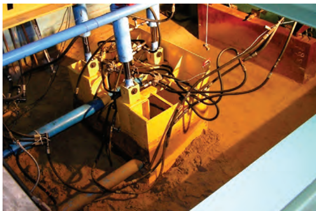
Грунтовый лоток
