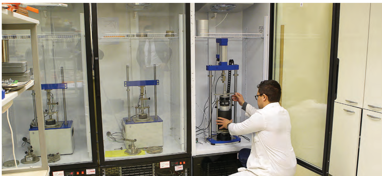
Комплект оборудования для испытаний образцов грунта в условиях трехосного сжатия вертикальной нагрузкой
