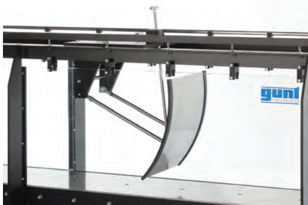
Сегментный затвор
