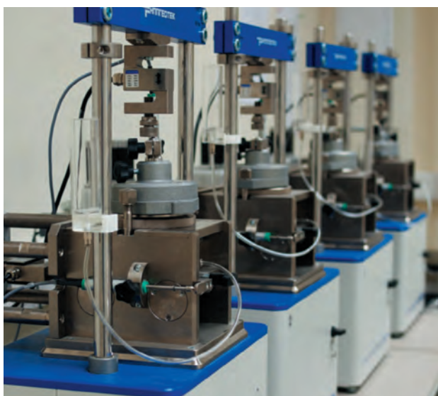
Оборудование для компрессионных испытаний
